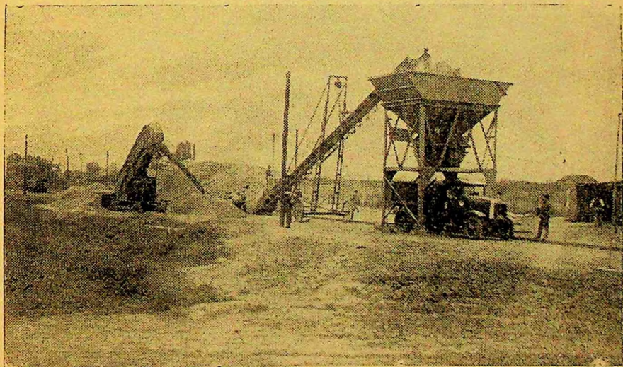
Bugnone, Guida y Cía. — Pavimentación. Camino Rosario-Timbúes, Ley 2157. Cargadores y Silo pesador de materiales
