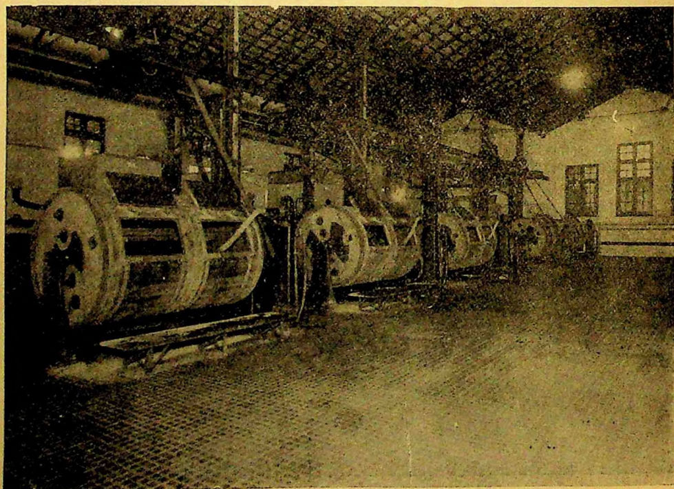
Fábrica de Manteca "Las Colonias", Rafaela. — Sala de batidores de manteca. The River Plate Dairy Co. Ltd.
