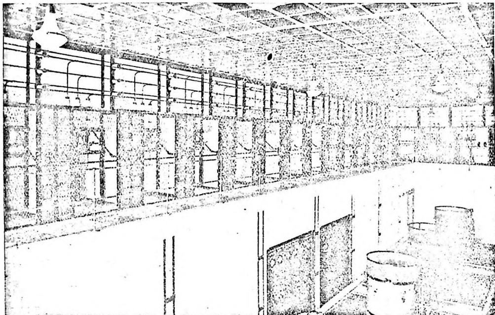
Vista interior de la Sub-Usina semi-automática a rectificadores de mercurio, instalada en el barrio Saladillo, de la Sociedad de Electricidad de Rosario
