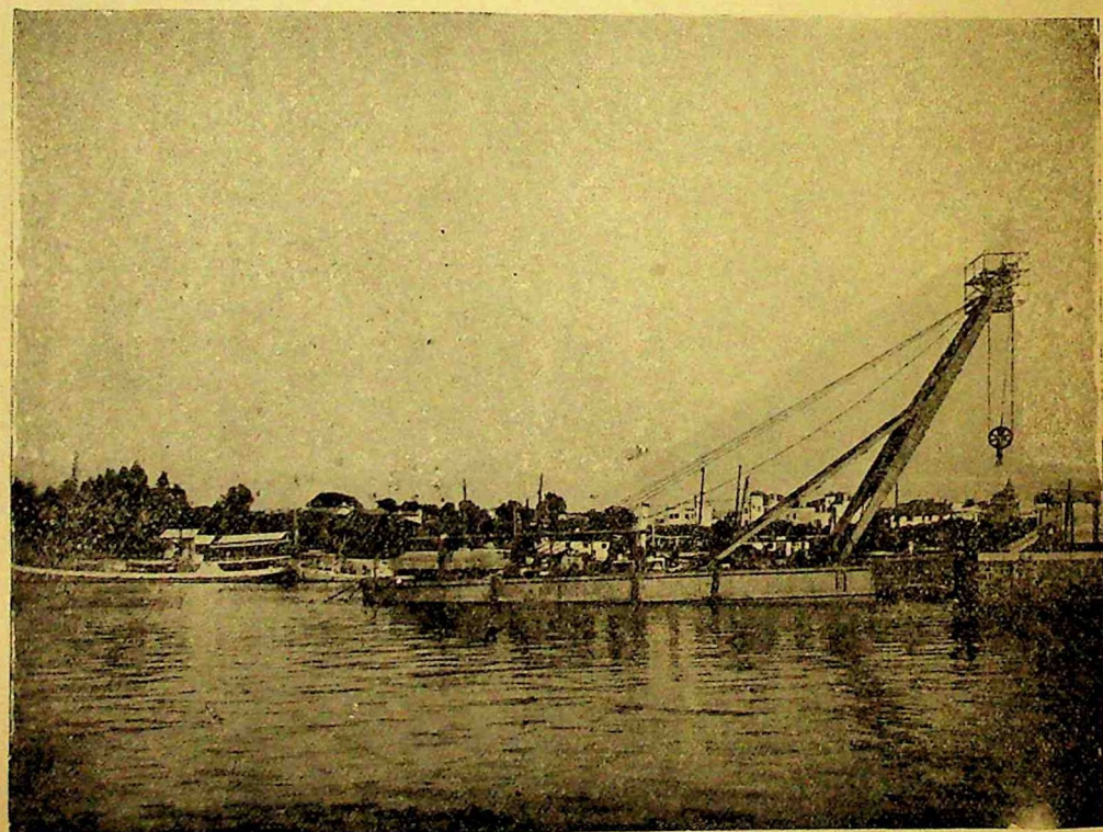
Grúa flotante de 55 toneladas del puerto de Rosario
