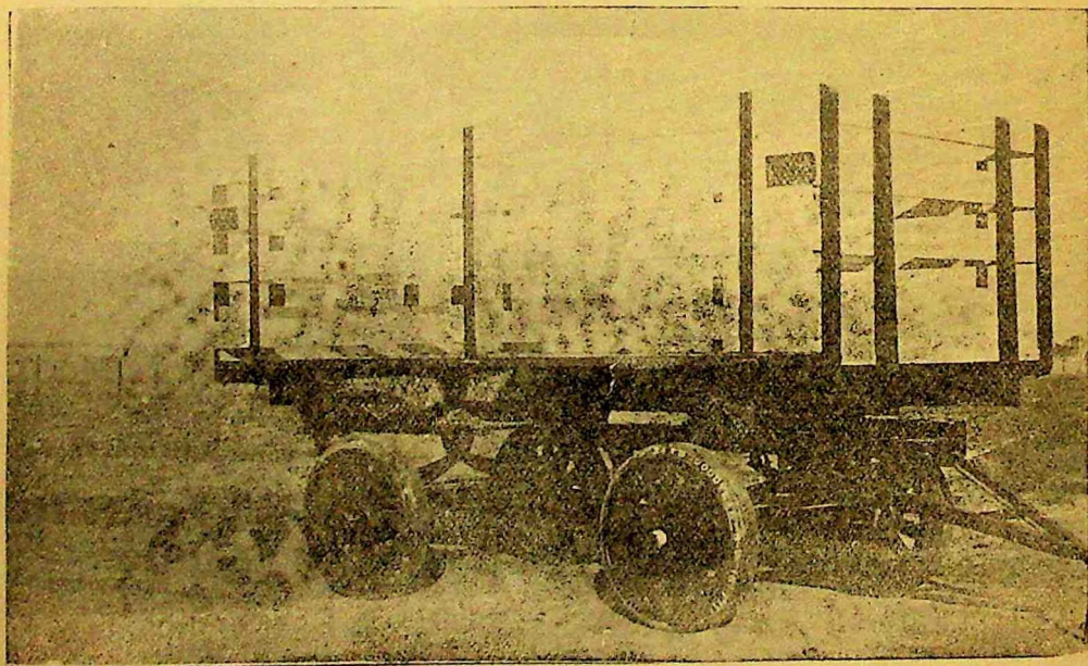
Acoplado especial con carrocería para transporte de nafta. — Fábrica de Acoplados y Anexos de Romagiale Hnos. — Cañada de Gómez.
