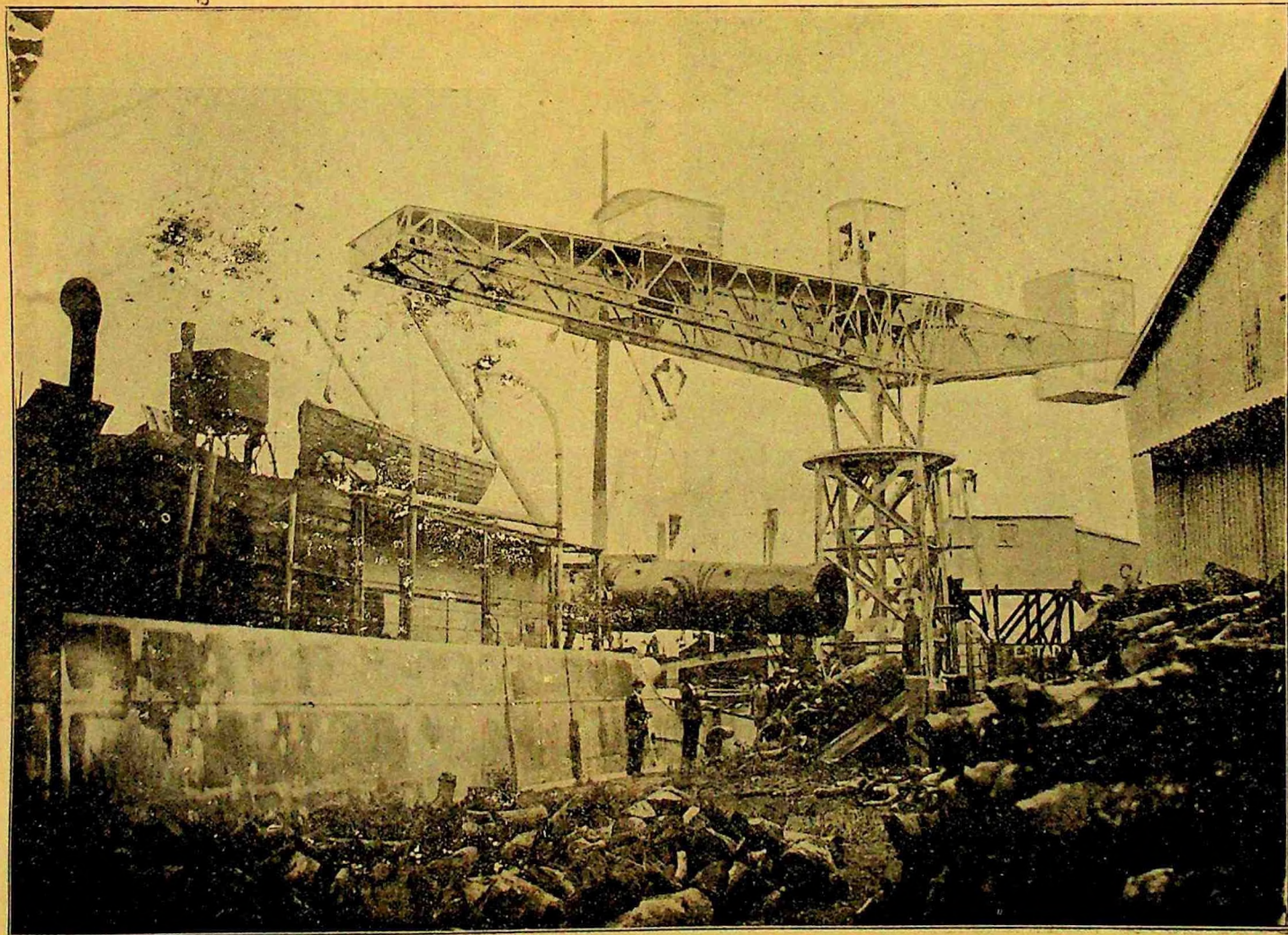
La poderosa grúa Titán. — Puerto de Santa Fe
