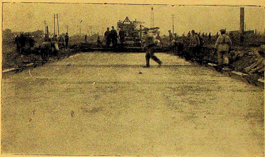
Bugnone, Guida y Cía. — Pavimentación. Camino Rosario-Timbúes, Ley 2157. Construcción de hormigón armado
