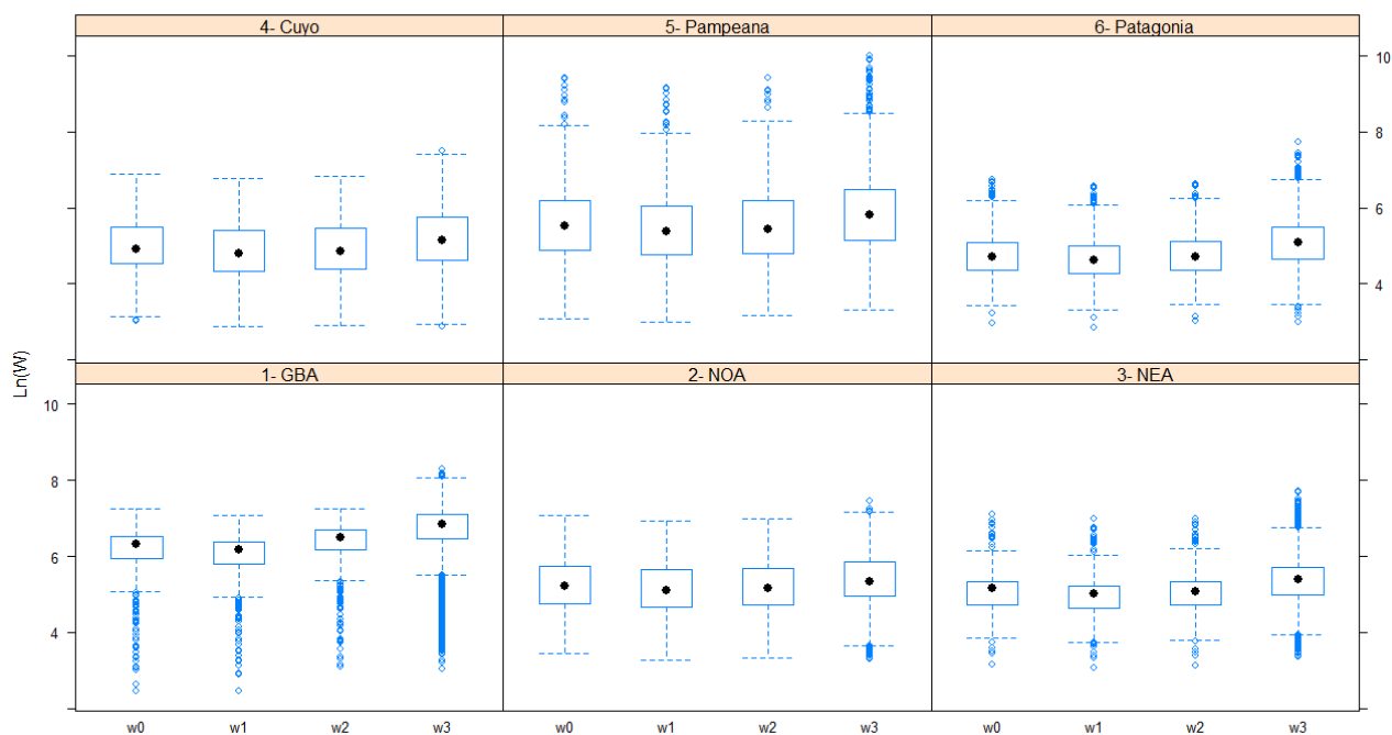
Gráfico 1. Distribución de las ponderaciones de los hogares, en escala logarítmica, según los distintos ajustes, por regiones
