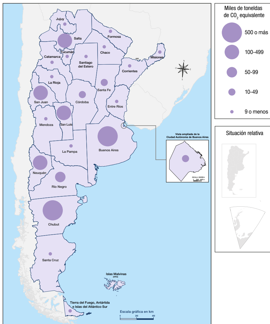
Mapa 24. Emisiones de gases de efecto invernadero del sector procesos industriales y uso de productos, por jurisdicción. Año 2022
