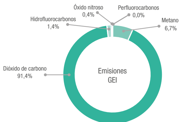
Gráfico 55. Generación de emisiones al aire de gases de efecto invernadero de Industria manufacturera, por tipo de gas. Año 2022
