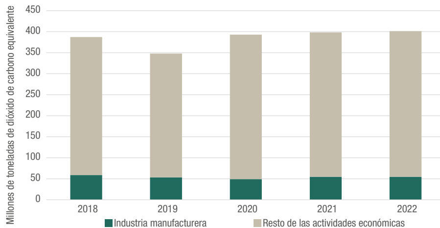
Gráfico 54. Generación de emisiones al aire de gases de efecto invernadero de Industria manufacturera. Años 2018-2022
