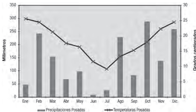
Gráfico 4. Precipitaciones y temperaturas medias mensuales por estación meteorológica de Posadas. Año 2012
