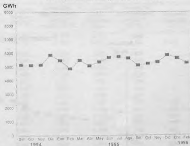
Energía eléctrica generada bruta
