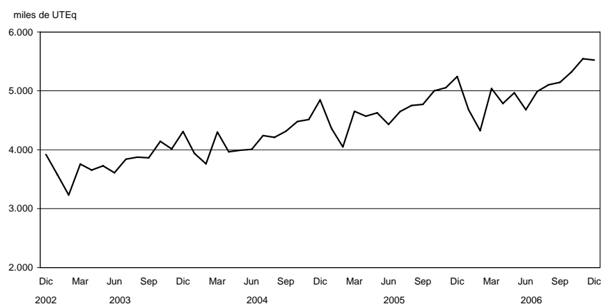
Gráfico 2.1.5.6 Vehículos pasantes por puestos de peaje en el acceso Ricchieri a la Ciudad de Buenos Aires
