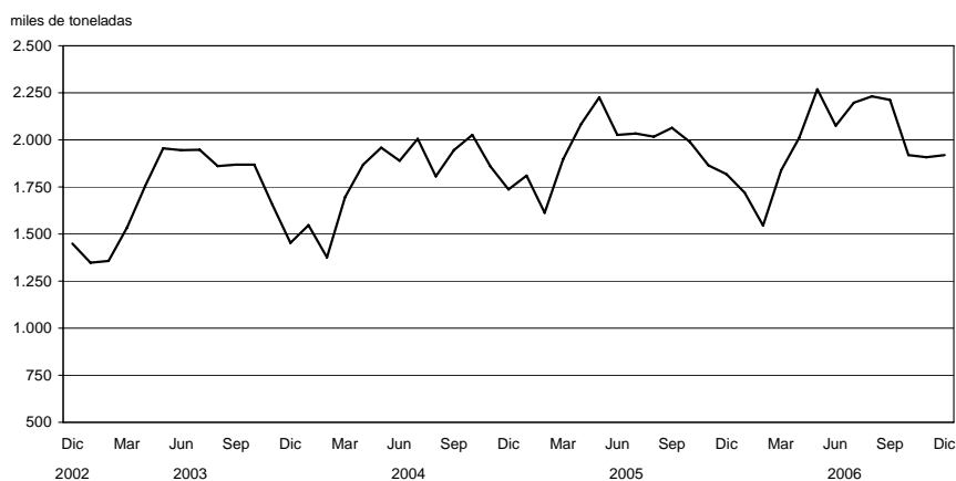
Gráfico 2.1.4.1 Carga transportada en el servicio ferroviario
