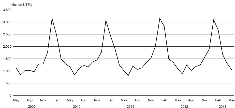
Gráfico 2.1.5.2 Vehículos pasantes por puestos de peaje en rutas de la provincia de Buenos Aires
