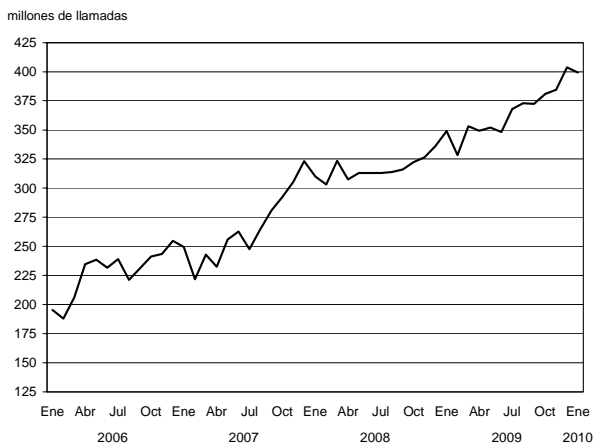
Gráfico 2.1.6.3 Llamadas interurbanas
