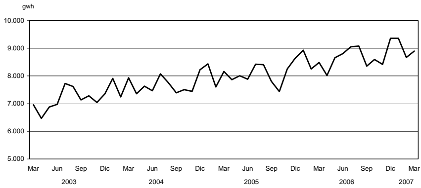
Gráfico 2.1.2.1 Generación neta de energía eléctrica
