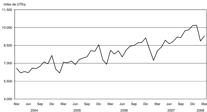
Gráfico 2.1.5.5 Vehículos pasantes por puestos de peaje en el acceso Oeste a la Ciudad de Buenos Aires
