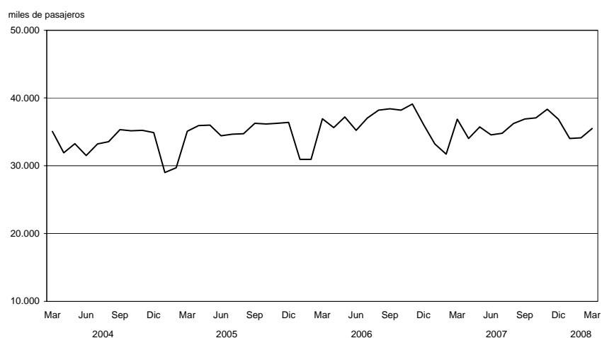
Gráfico 2.1.3.1 Pasajeros transportados en ferrocarriles urbanos
