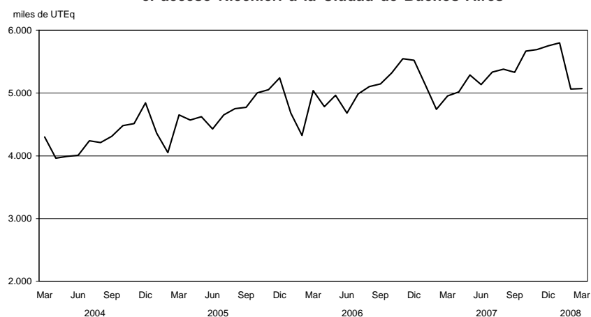
Gráfico 2.1.5.6 Vehículos pasantes por puestos de peaje en el acceso Ricchieri a la Ciudad de Buenos Aires
