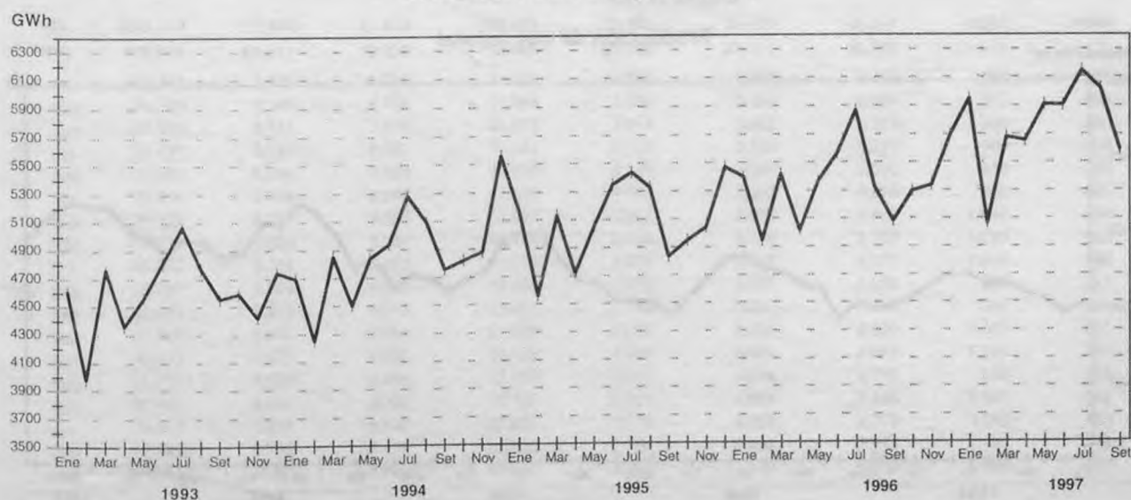
Oferta interna de energía eléctrica
