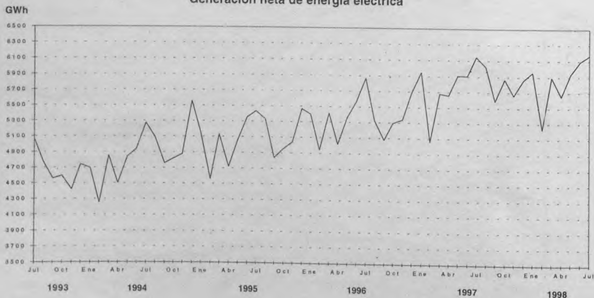
Generación neta de energía eléctrica
