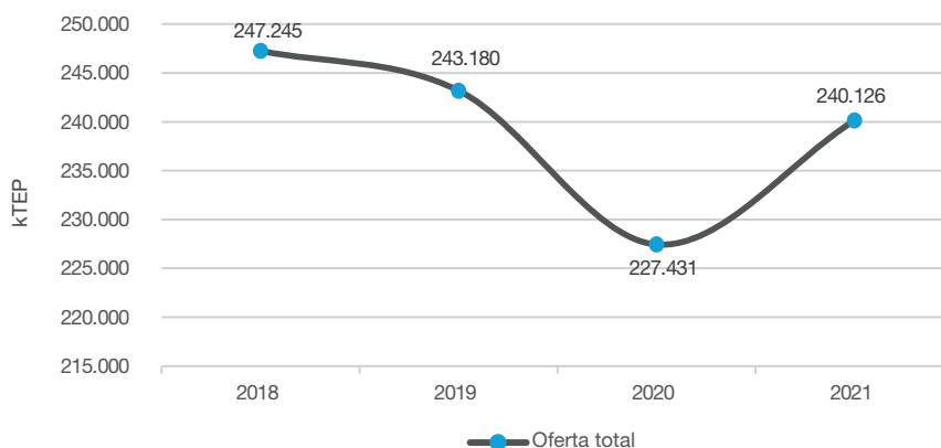
Gráfico 7. Oferta energética total. Total del país. Años 2018-2021
