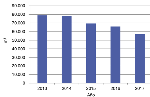
Producción de tableros compensados
