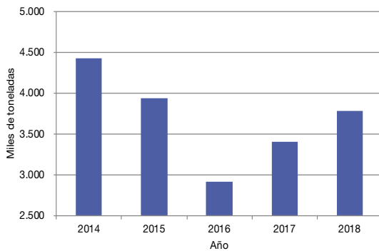
Producción de hierro primario
