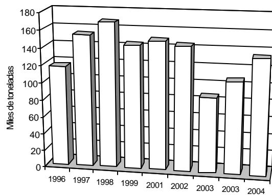
Producción de hierro redondo para hormigón Acumulado Ene-Abr
