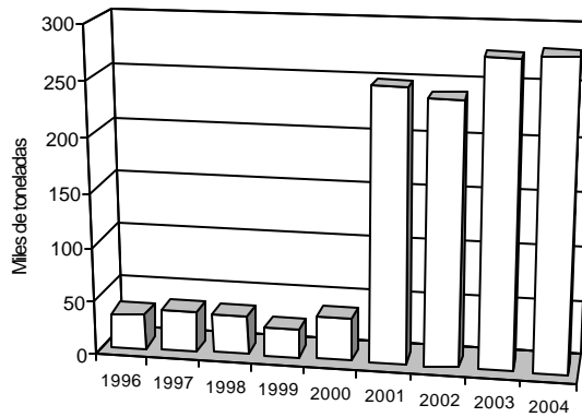
Producción de amoníaco Acumulado Ene-Abr
