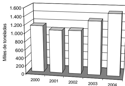
Producción de laminados no planos en caliente Acumulado Ene-Dic
