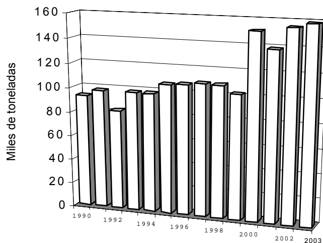
Producción de aluminio primario Acumulado Ene - Jul
