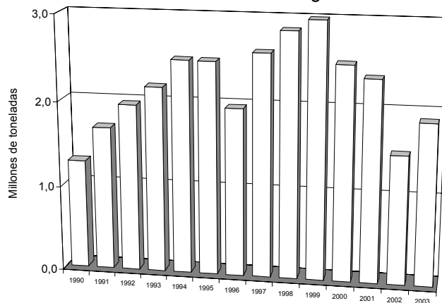
Producción de cemento portland Acumulado Ene - Jun
