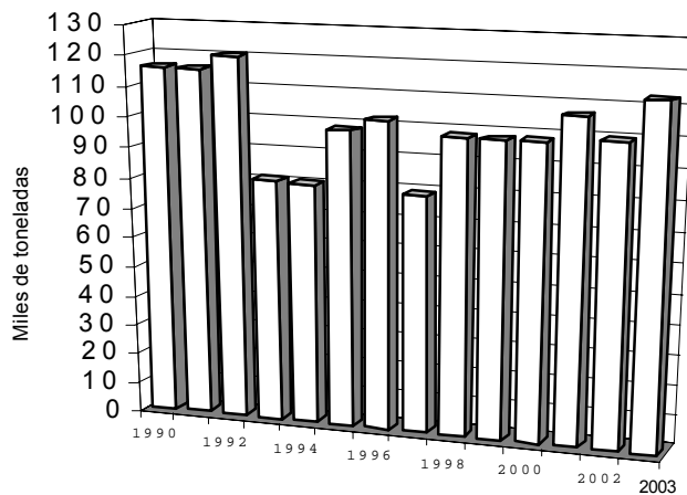
Producción de papel para diarios Acumulado Ene - Jul
