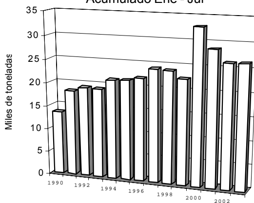
Producción de hilados sintéticos Acumulado Ene - Jul
