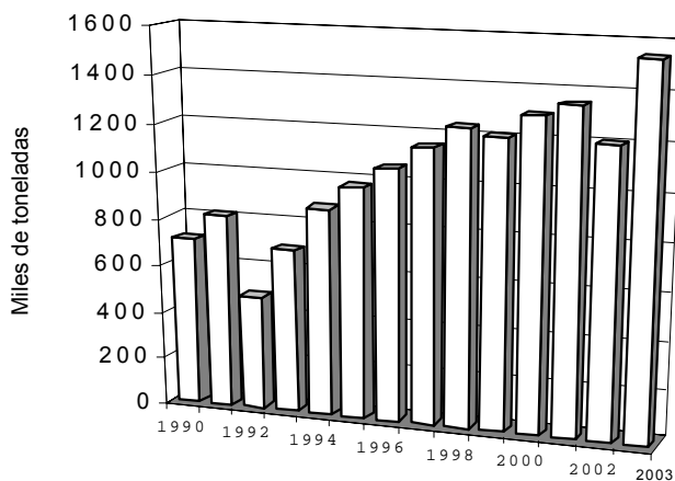
Producción de laminados no planos en caliente Acumulado Ene - Jul
