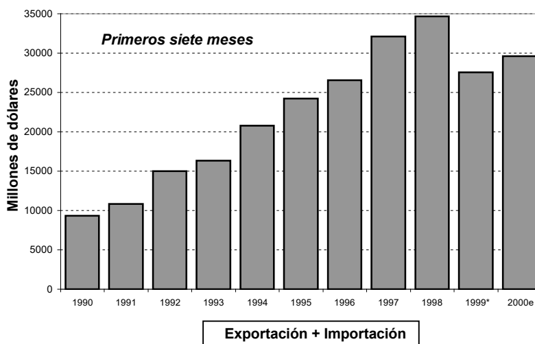
Gráfico 1 - Intercambio Comercial
