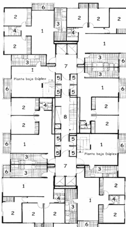
Planta tipo
