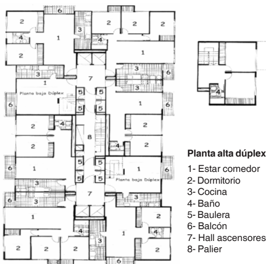
Planta tipo
