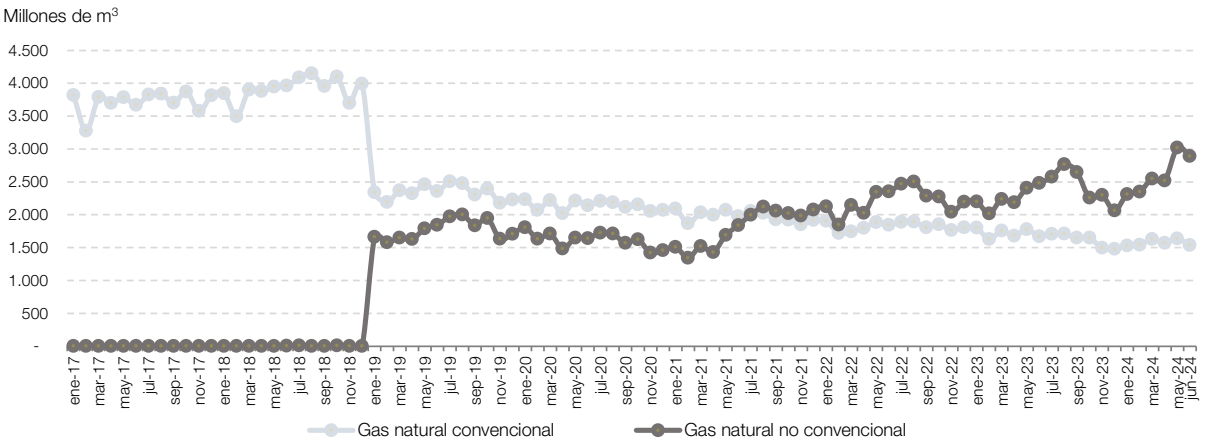
Gráfico 7.2 Extracción de gas natural convencional y no convencional, en millones de m³. Enero 2017-junio 2024
