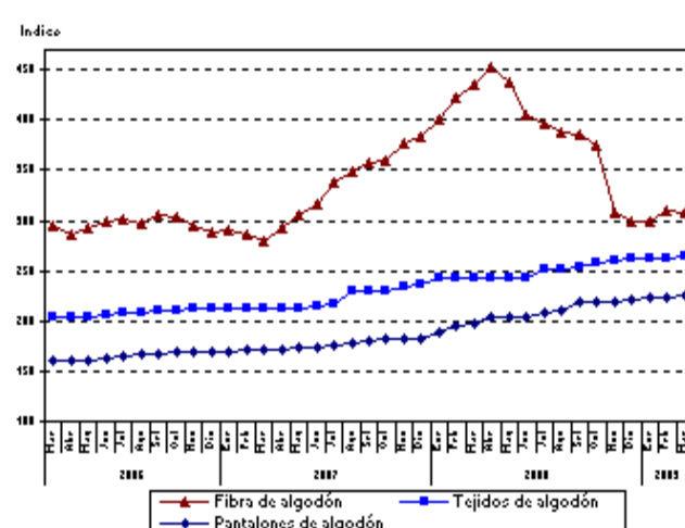
Evolución de los índices de Fibra algodón, Tejidos de algodón y Pantalones de algodón, IPIB base 1993=100
