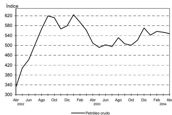
Petróleo crudo
