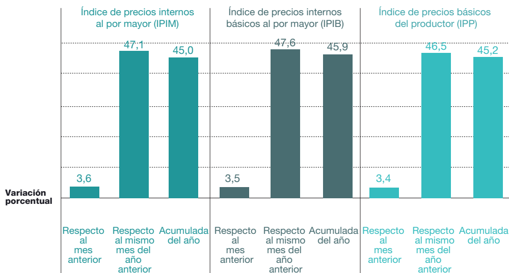
Gráfico 1. Sistema de índices de precios mayoristas. Variación porcentual. Octubre de 2019*
