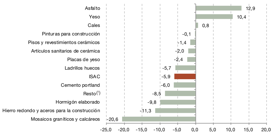
Gráfico 2. Insumos para la construcción. Serie original base 2004=100, en variación porcentual interanual. Agosto de 2019
