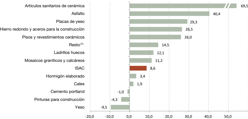
Gráfico 2. Insumos para la construcción. Serie original base 2004=100, en variación porcentual interanual. Mayo de 2025
