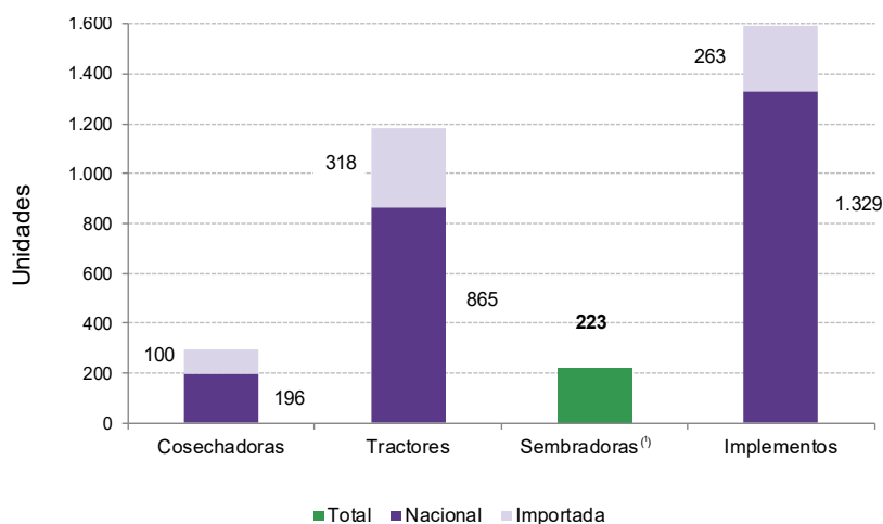
Gráfico 1. Venta de maquinaria agrícola nacional e importada, en unidades. Primer trimestre de 2019 e
